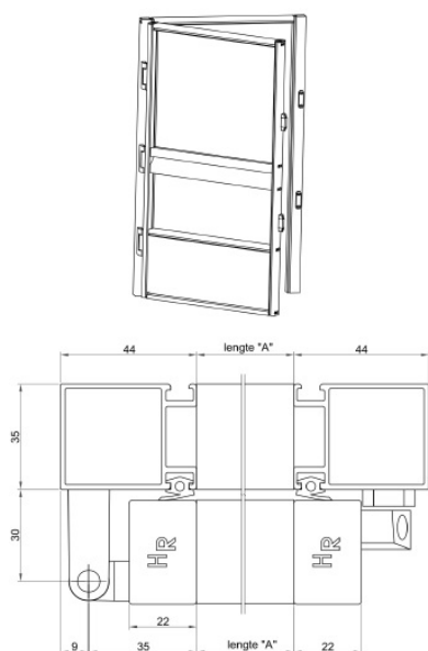
Cadre et vue du dessus
