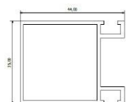
PROFIL DE CADRE DORMANT (HR051) : 44 x 35 MM LONGUEUR PROFIL : 4,5 M
